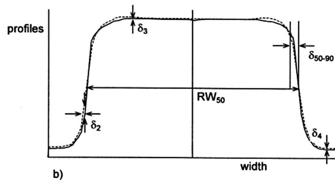
شکل ۱- نواحی مختلف موجود در توزیع دوز و کمیت های مربوط به آنها (a) بر روی درصد دوز عمقی و (b) بر روی پروفایل بیم تابشی
